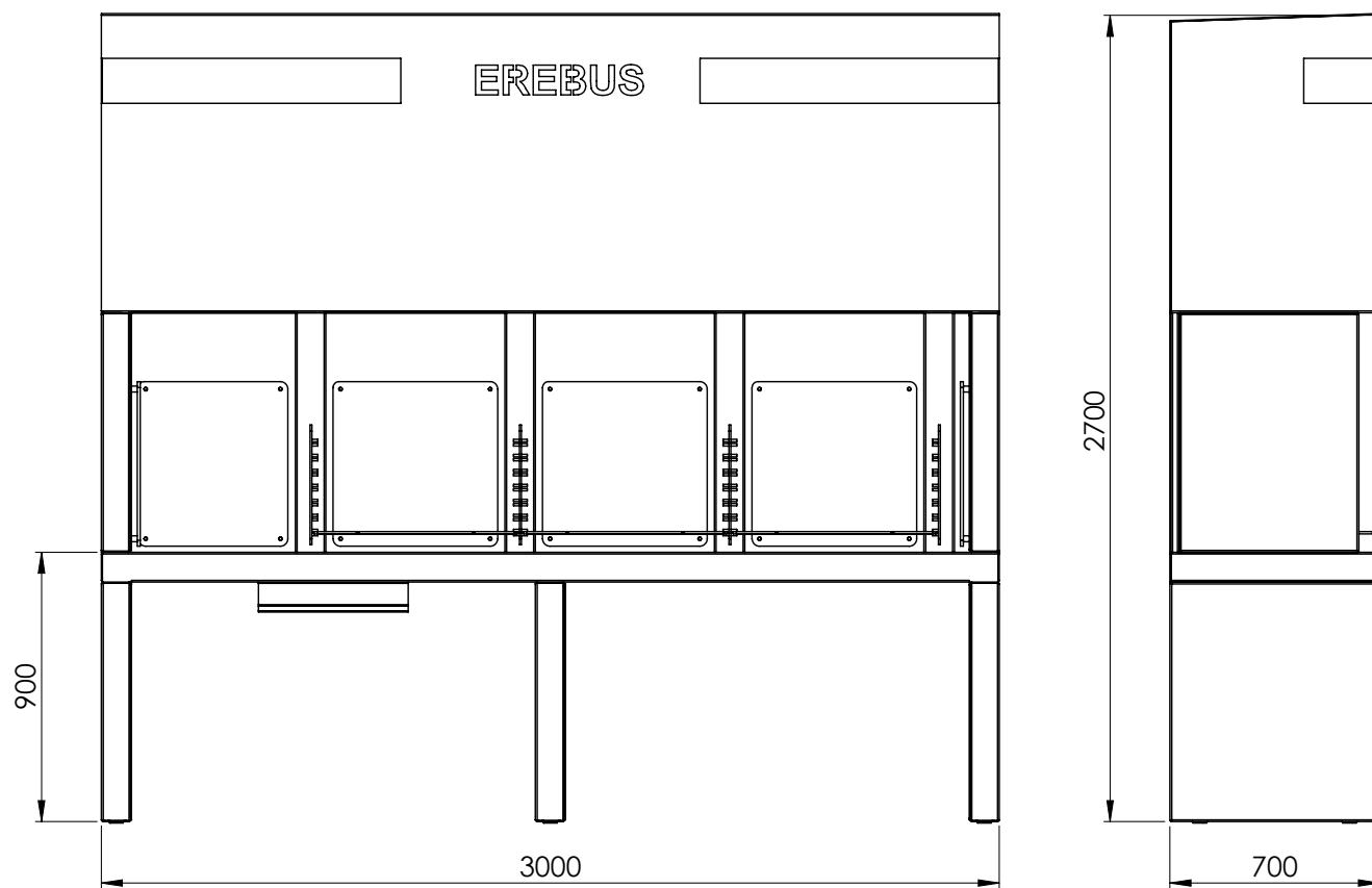
Medidas estándar de la barbacoa (mm).
