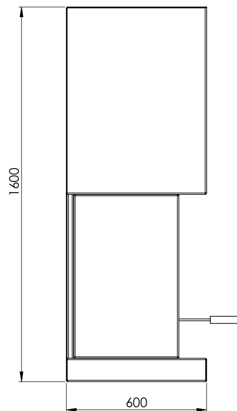
Medidas estándar de la barbacoa (mm).
