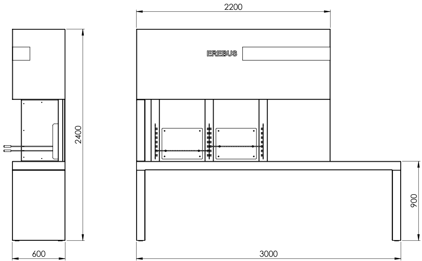
Medidas estándar de la barbacoa (mm).
