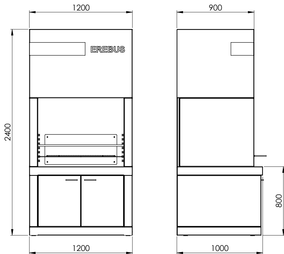
Medidas estándar de la barbacoa (mm).
