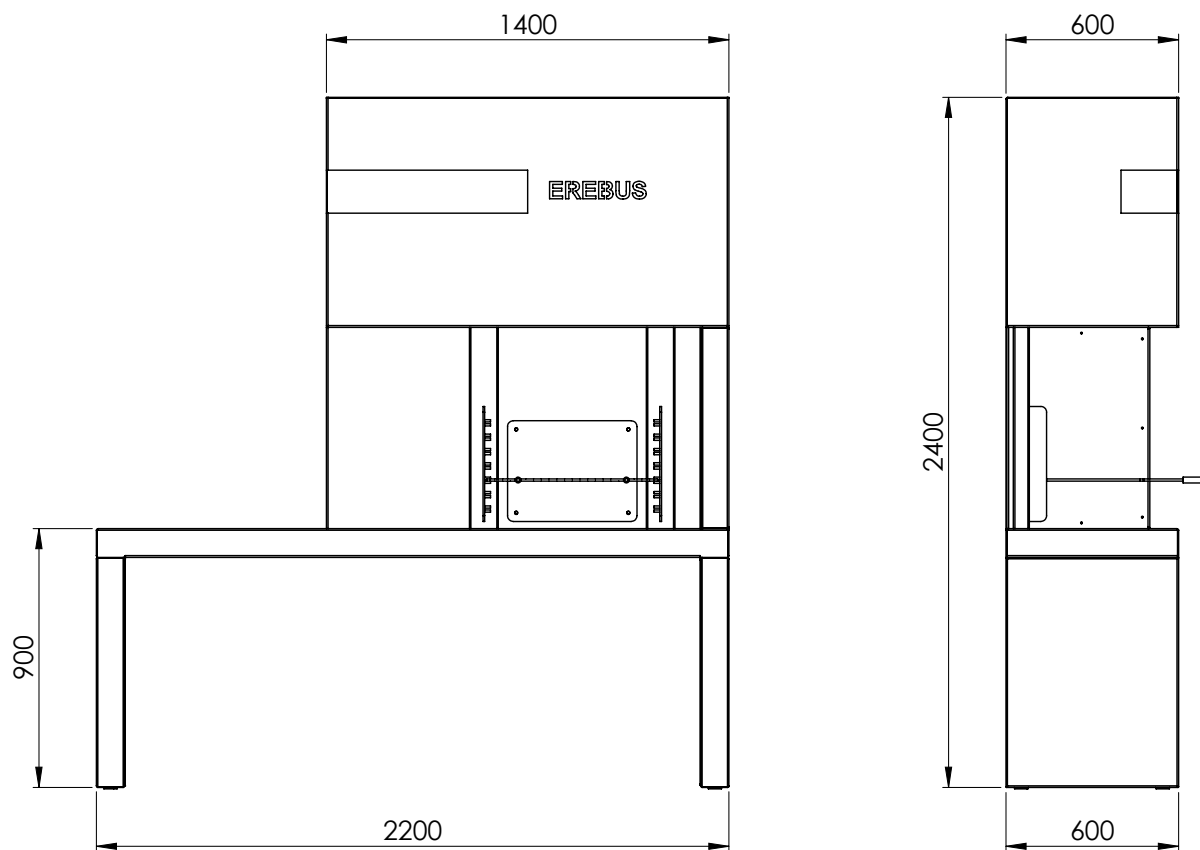
Medidas estándar de la barbacoa (mm).
